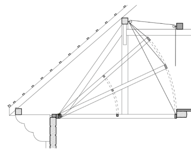
Panou termic izolatant reglabil (folie clară din polycarbonat)
