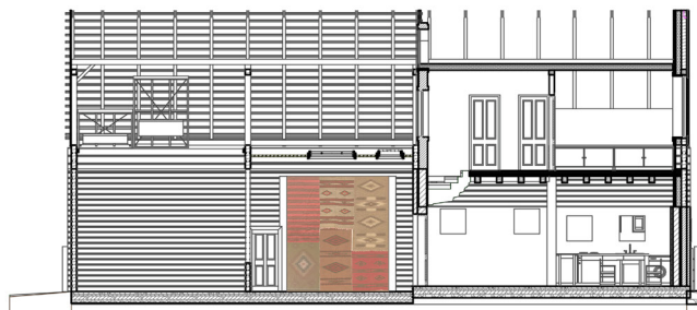
Dispunerea tavanului casetat
